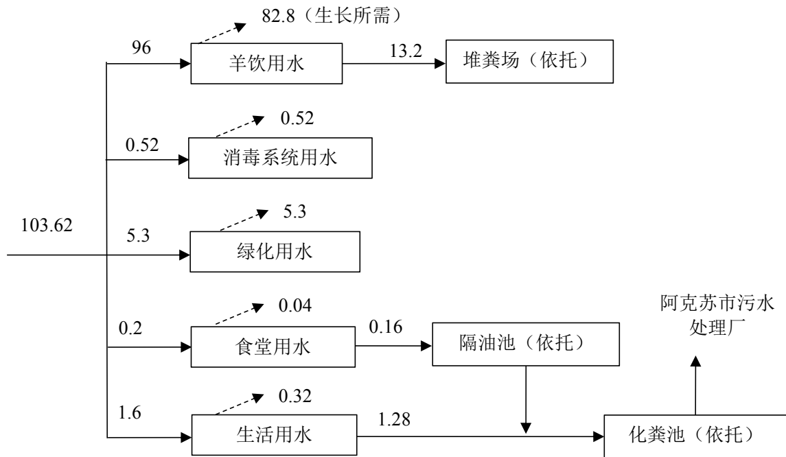
图 3.8-1 项目给排水平衡图（绿化季节，210 天） 单位：m³/d
