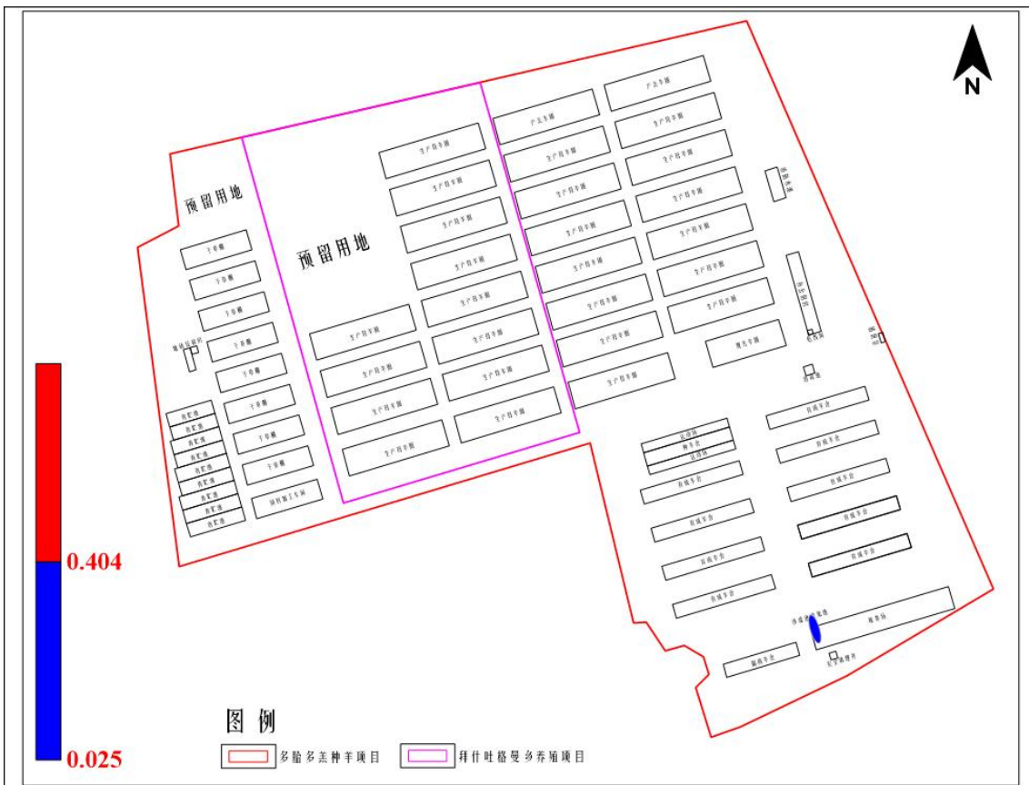
图 5.4-4 氨氮浓度随时间变化运移结果图（叠加背景值后）
