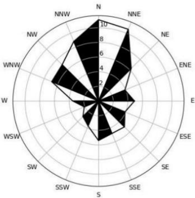
图 5.2-1 区域近 20 年风频玫瑰图
