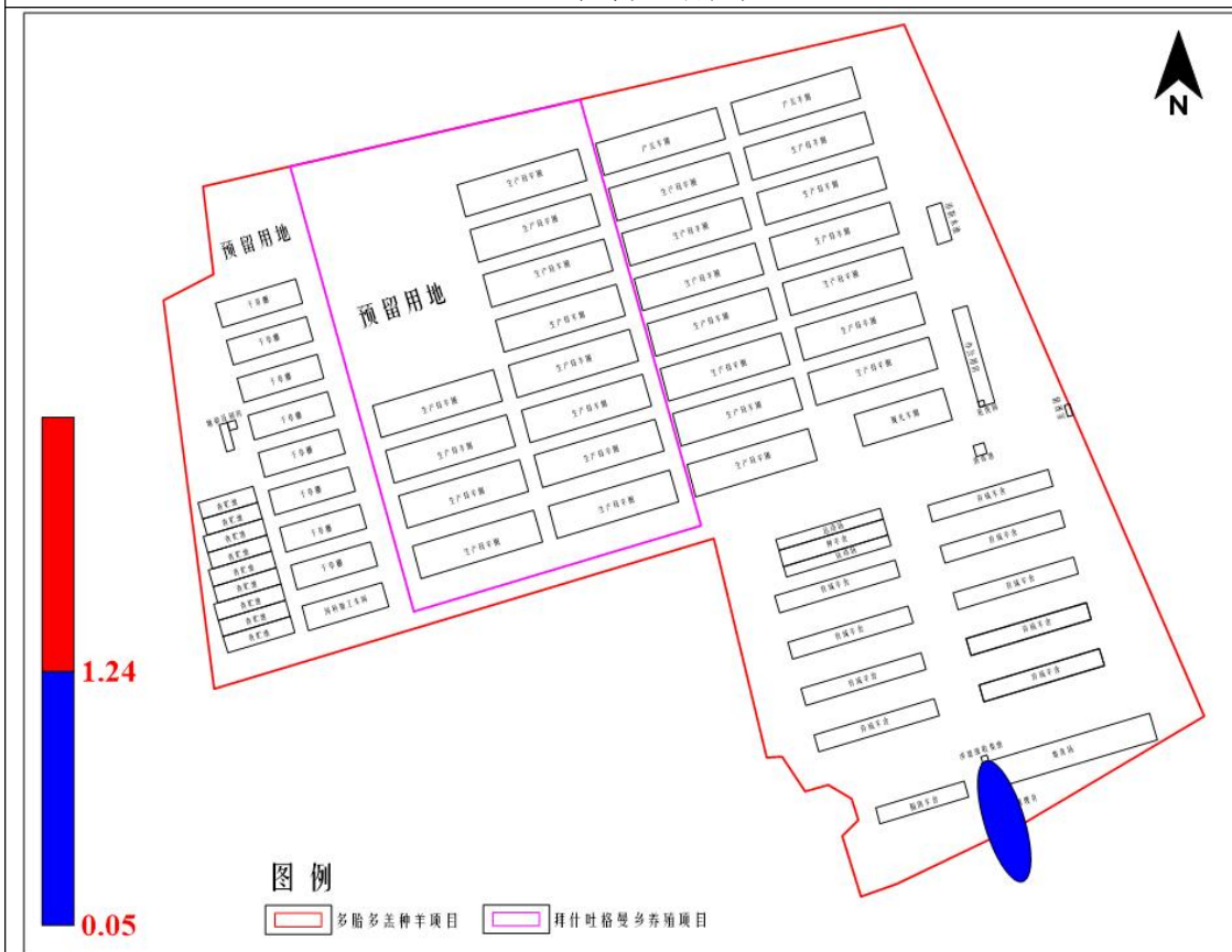
图 5.4-2 耗氧量浓度随时间变化运移结果图（叠加背景值后）
