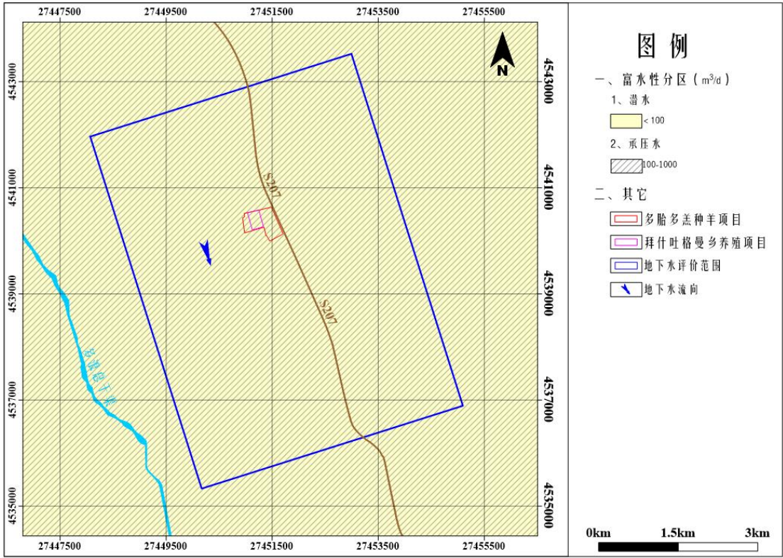
图 5.4-1 评价区水文地质图
