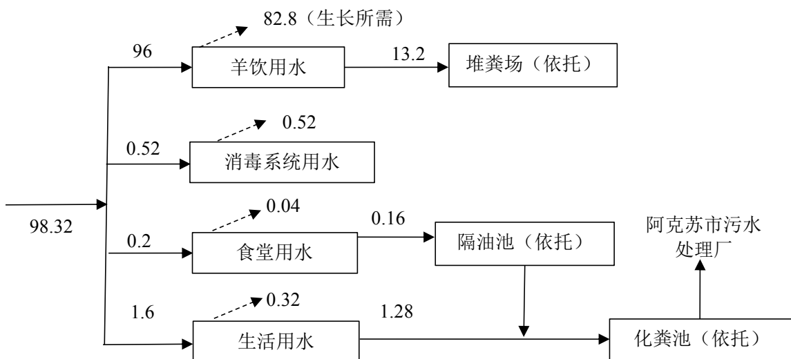
图 3.8-1 项目给排水平衡图（绿化季节，210 天） 单位：m³/d
