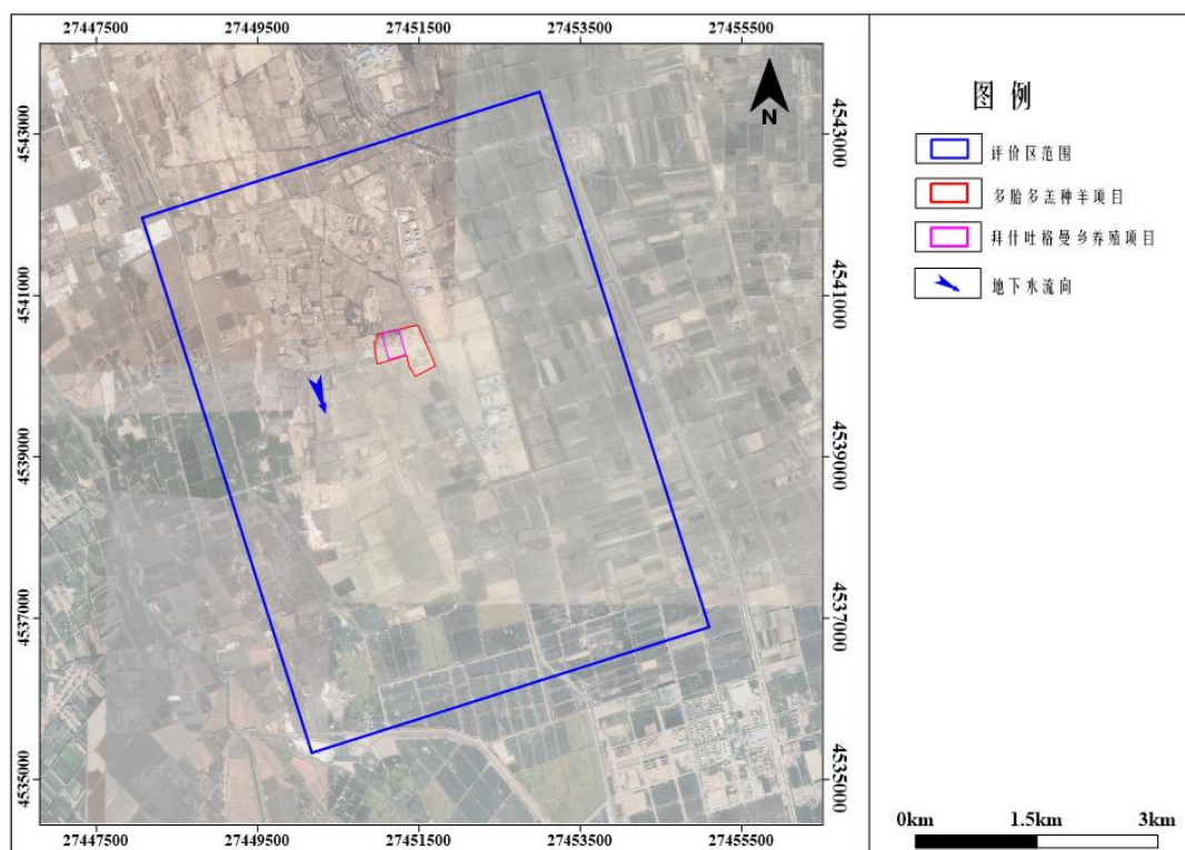
图 2.4-1 地下水调查评价范围示意图
