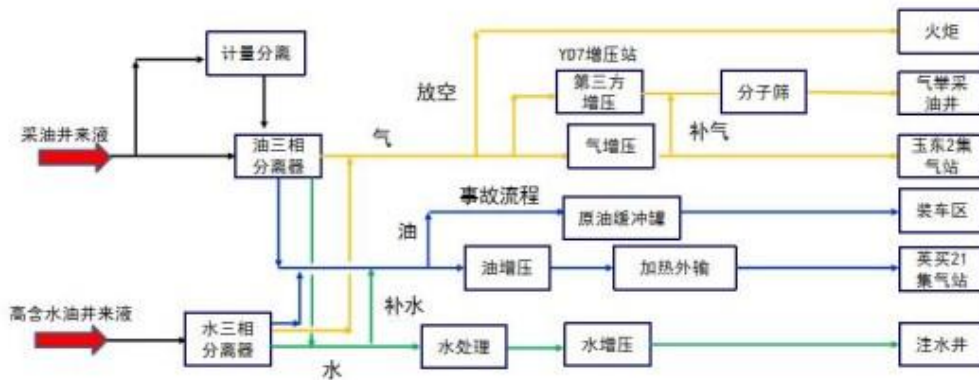
图 3.1-1 英买处理厂工艺流程图
