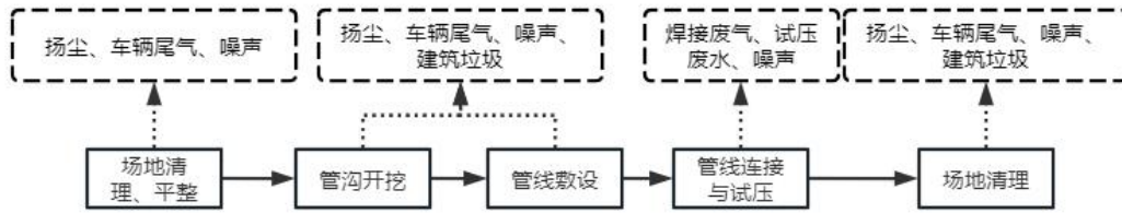
图 3.3-4 管道工程施工阶段工艺流程图
