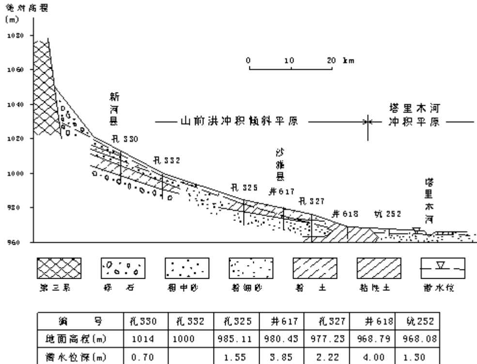
图 5.3-2 水文地质剖面示意图
