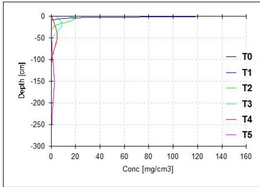
图 5.6-2 石油烃在不同时间沿土壤垂向迁移情况
