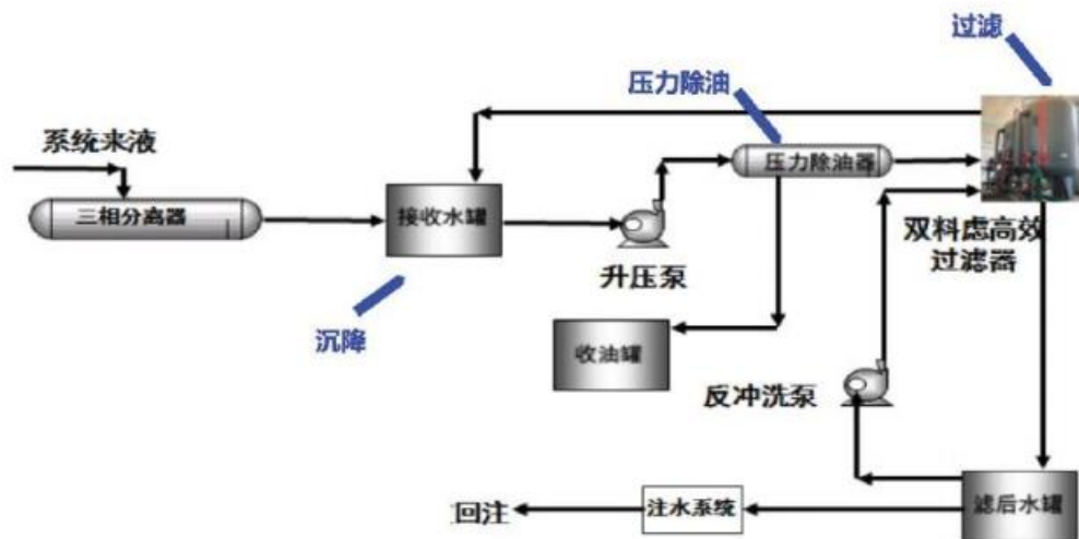
图 3.2-5 英潜油气运维中心污水处理工艺流程图
