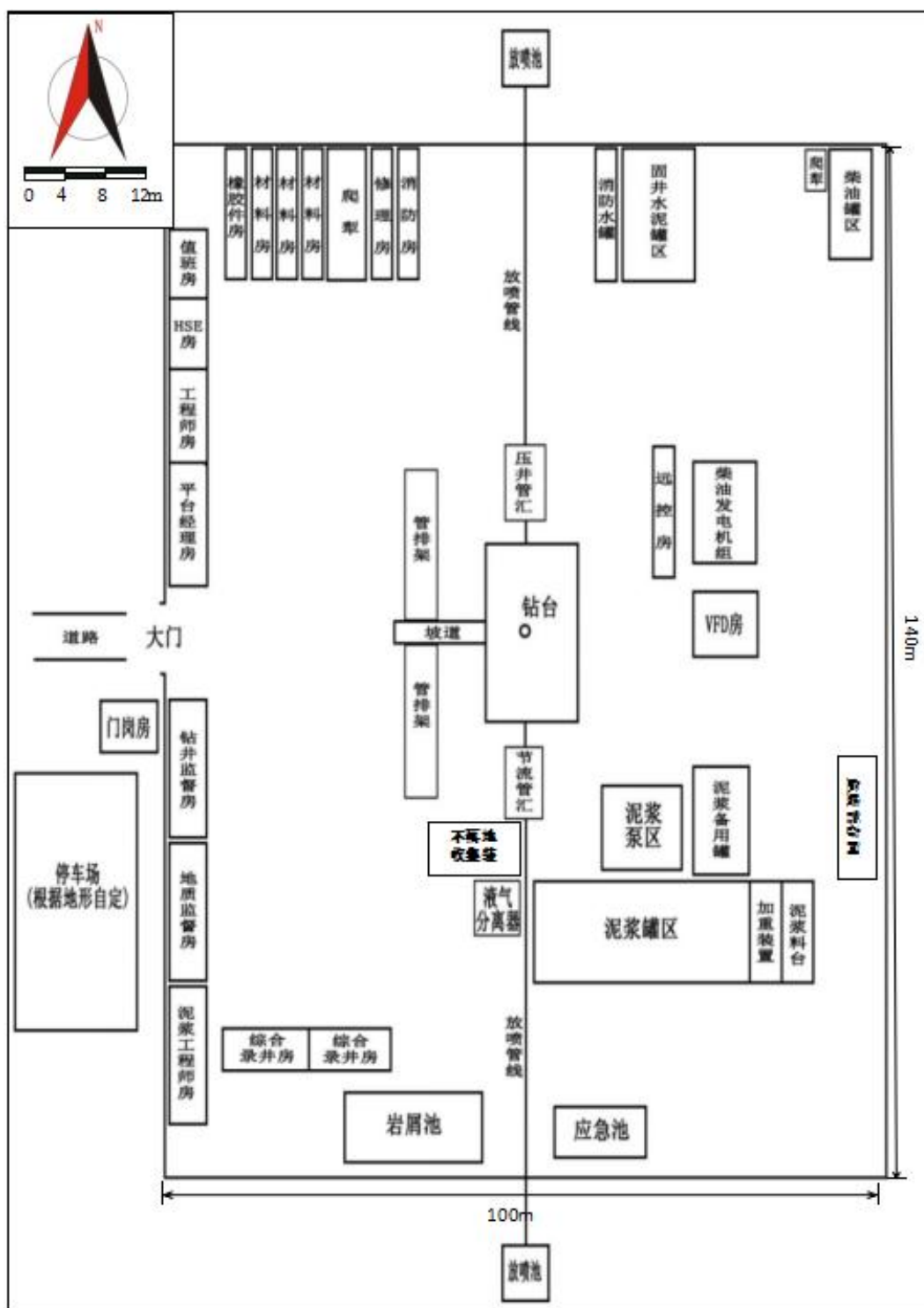
图 3.2-3 祥探 1 井场平面布置图
