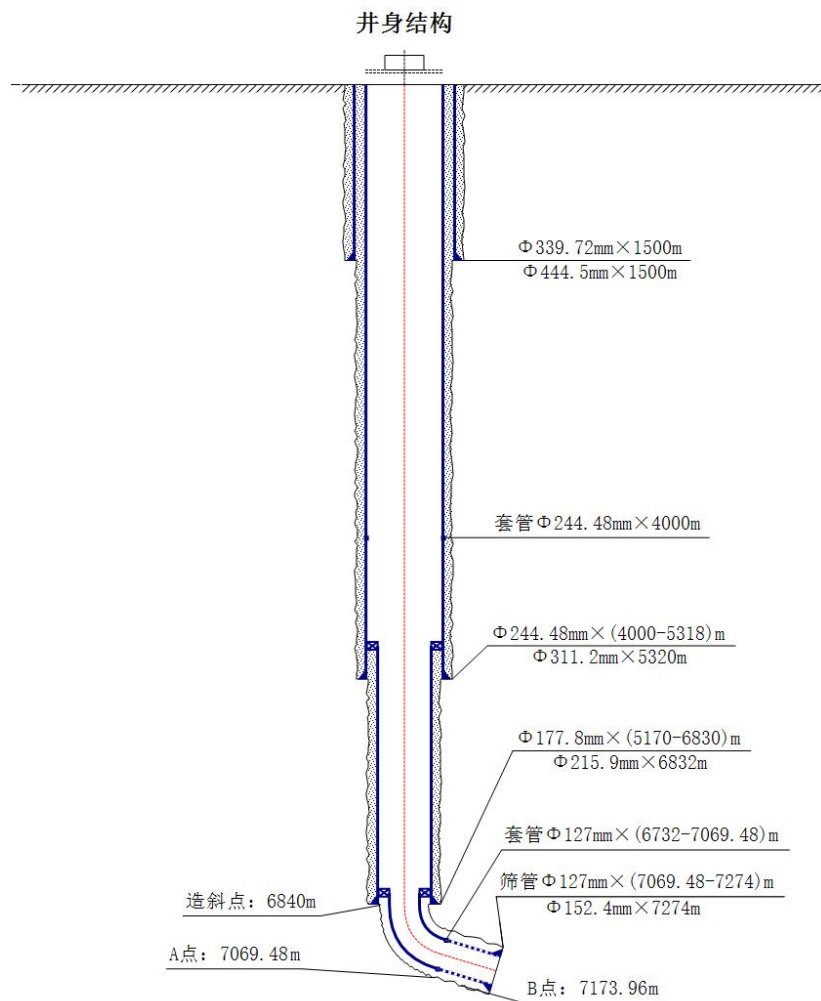
图 3.2-2 祥探 1 井井身结构
