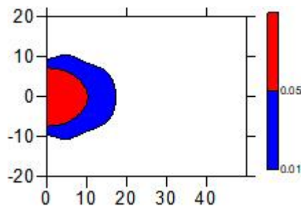
(1) 100d 时污染晕运移分布图
