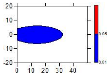
(2) 1000d 时污染晕运移分布图
