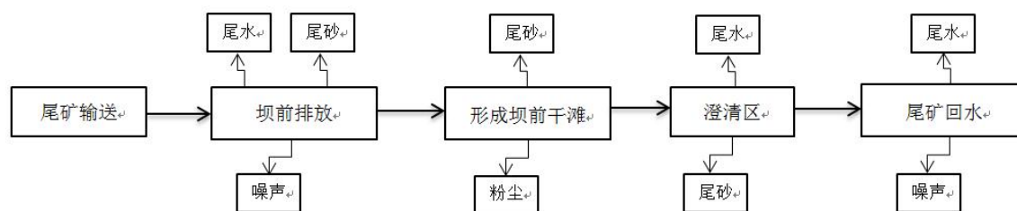
图 3.2-4 运行期产污环节示意图
