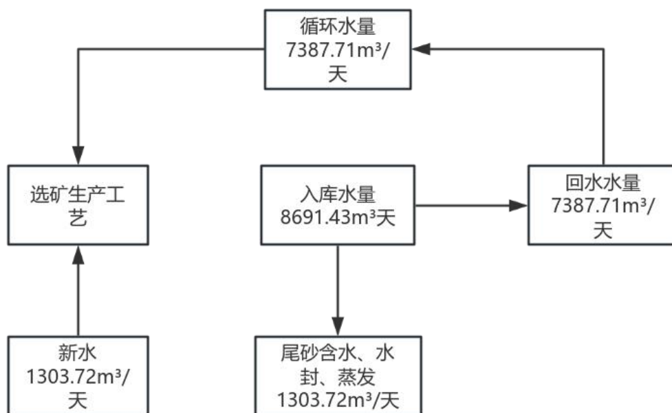
图 3.2-1 尾矿库水平衡图
