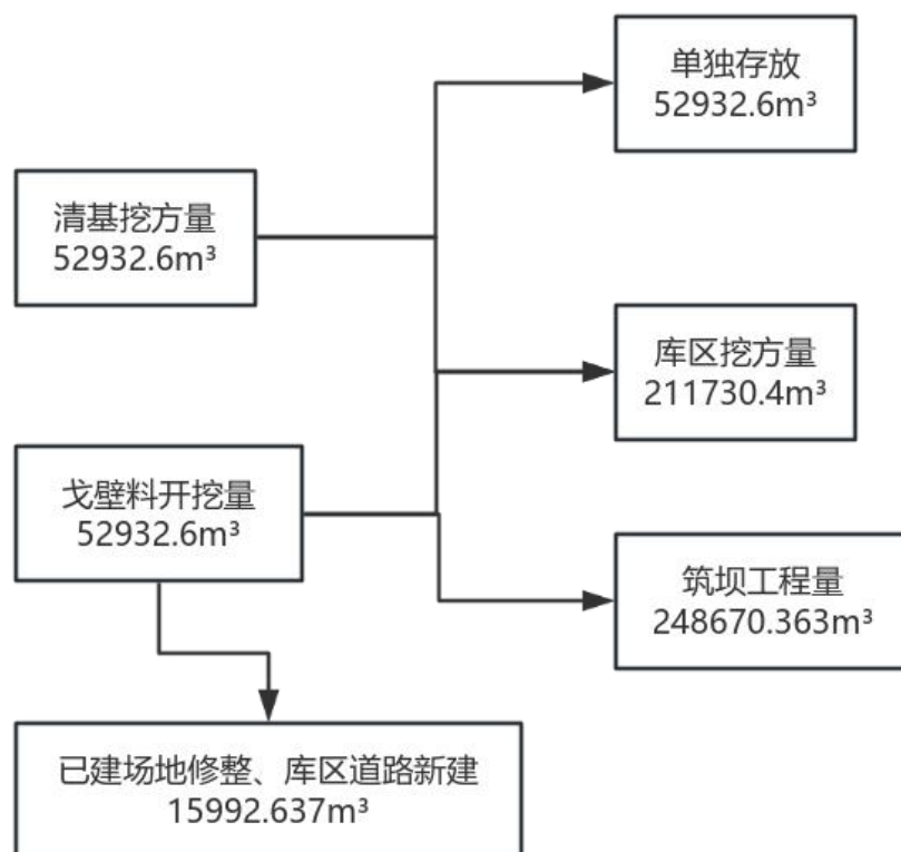
图 3.2-2 土石方平衡图
