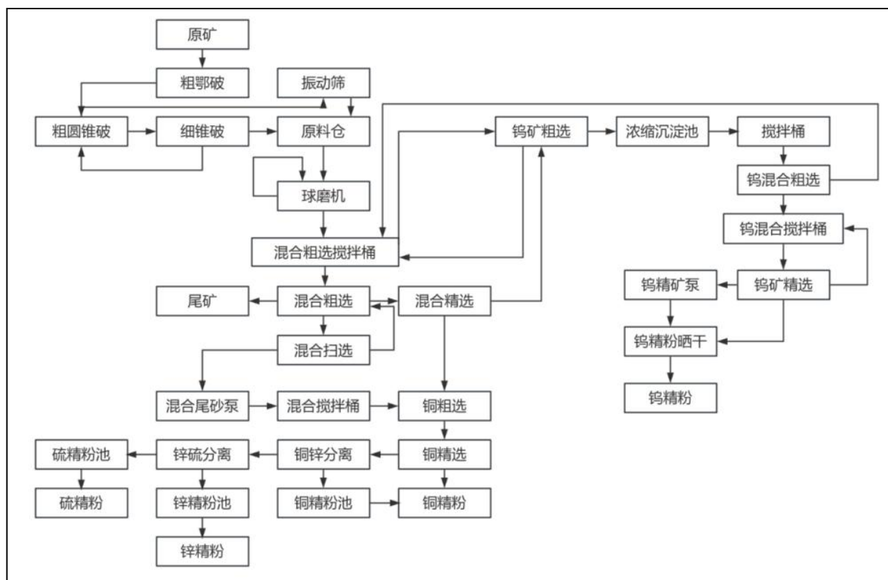
图 3.1-2 选矿厂工艺流程图
