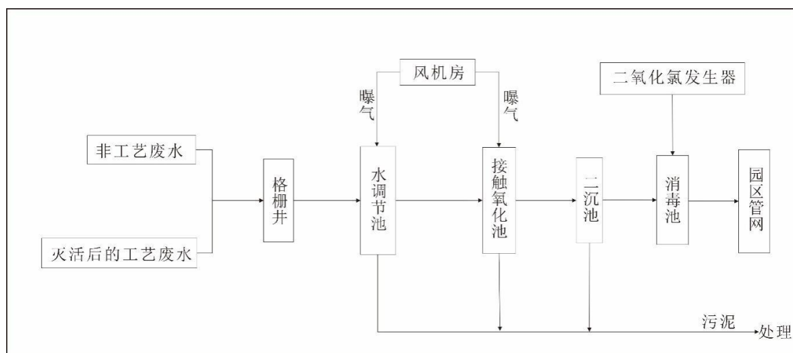
图 3.1-8 污水处理站处理工艺流程图
