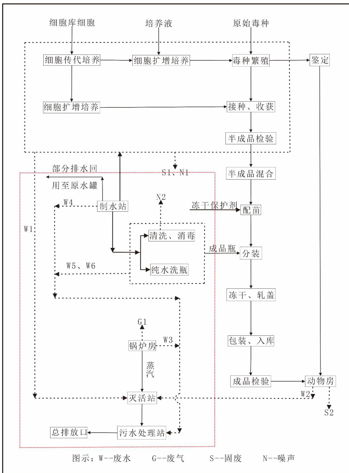
图 3.1-2 细胞（病毒）活疫苗生产线工艺流程及产污节点图
