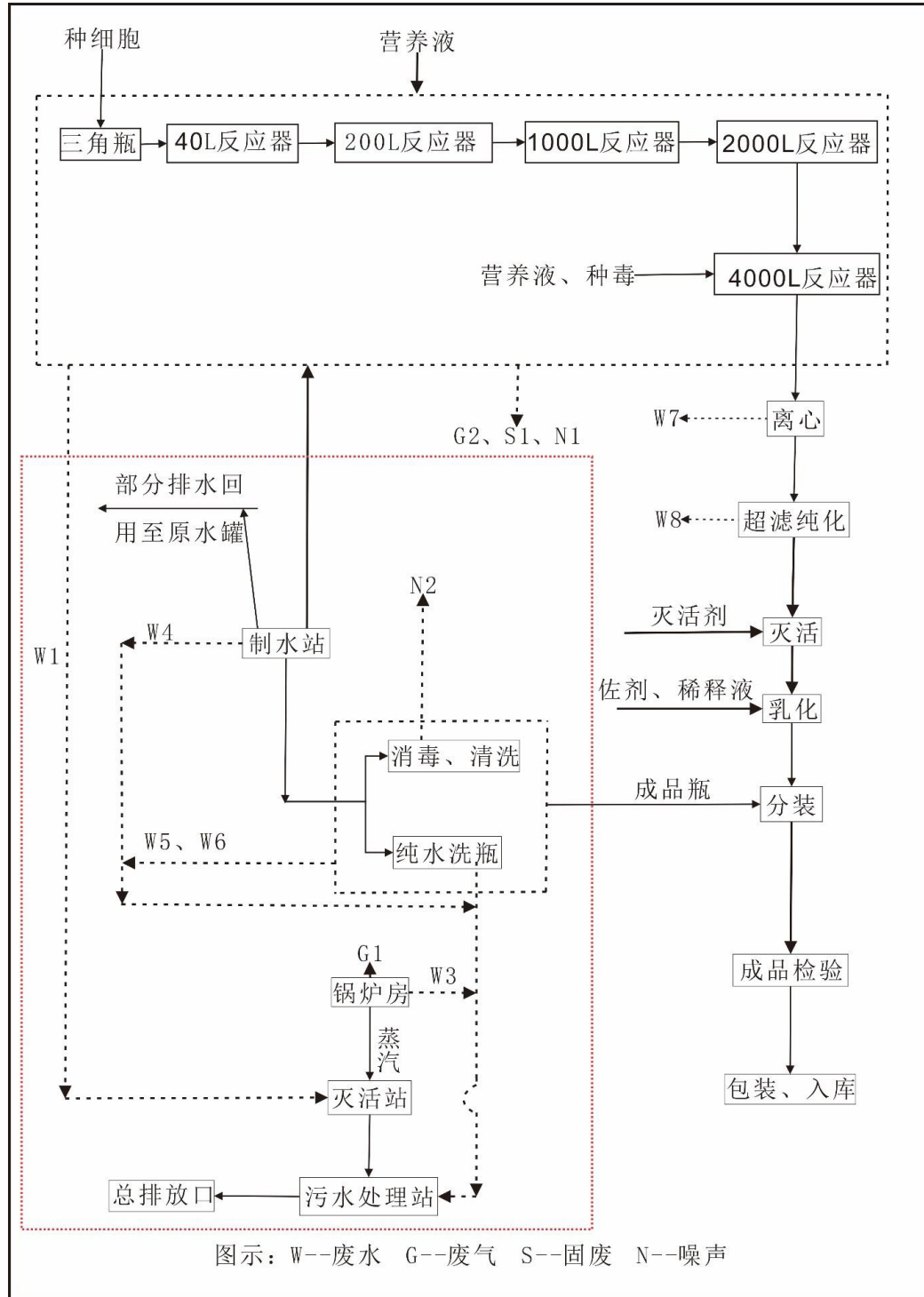
图 3.1-6 细胞培养病毒灭活疫苗生产线工艺流程及产污节点图
