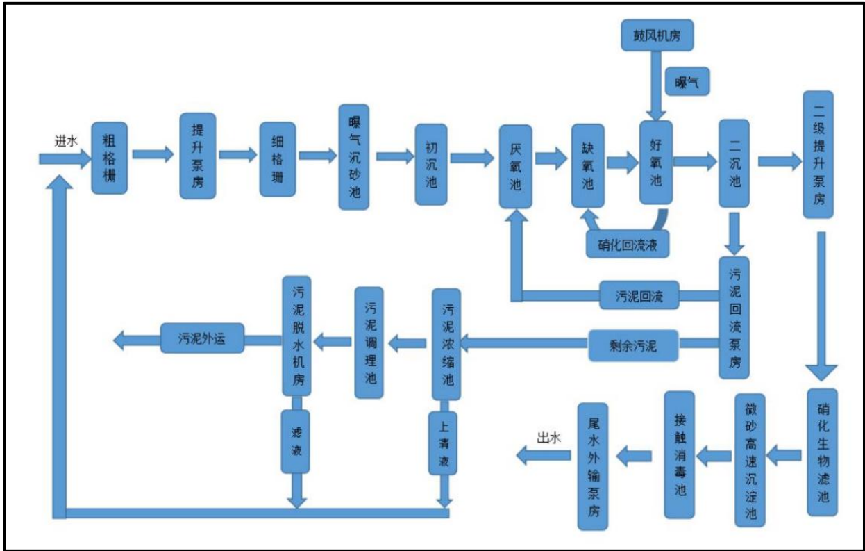
图 6.2-2 污水处理厂处理工艺流程图
