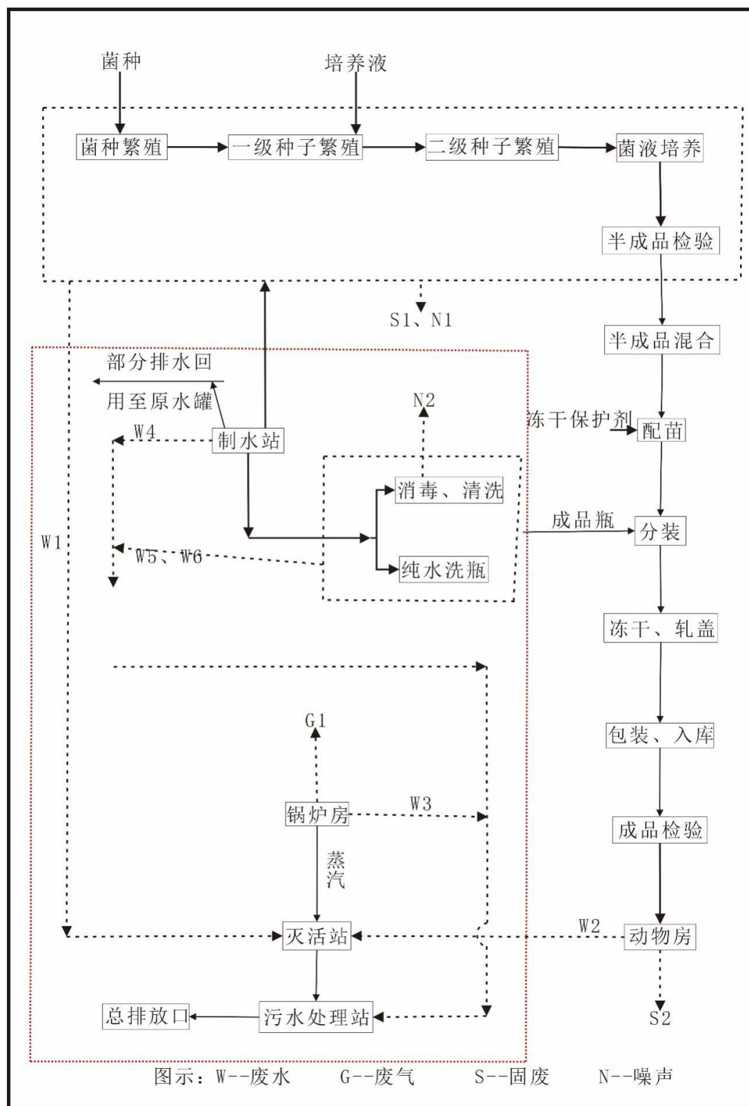
图 3.1-3 布氏菌病活疫苗生产线工艺流程及产污节点图
