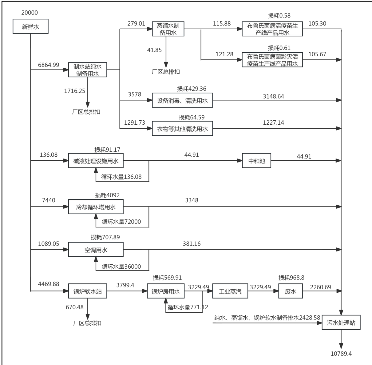
图 3.2-1 本项目水平衡图 单位: m³/a
