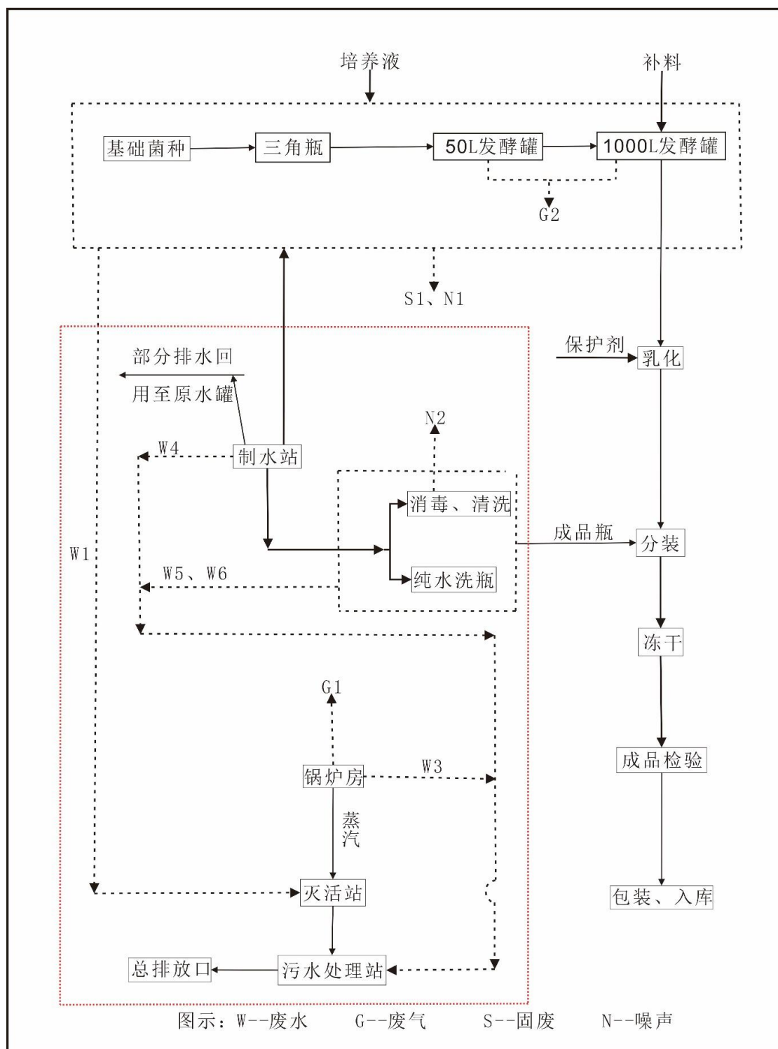
图 3.1-5 炭疽芽孢活疫苗生产线工艺流程及产污节点图
