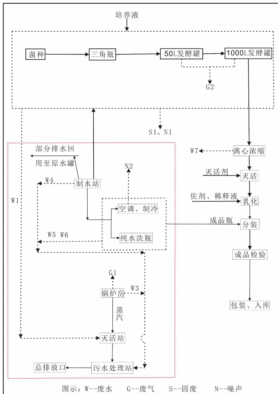
图 3.1-4 细菌灭活疫苗（含细菌培养亚单位疫苗）和梭菌灭活疫苗 生产线工艺流程及产污节点图
