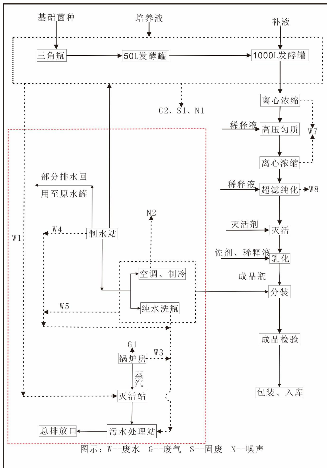
图 3.1-7 细胞悬浮培养病毒灭活疫苗生产线工艺流程及产污节点图
