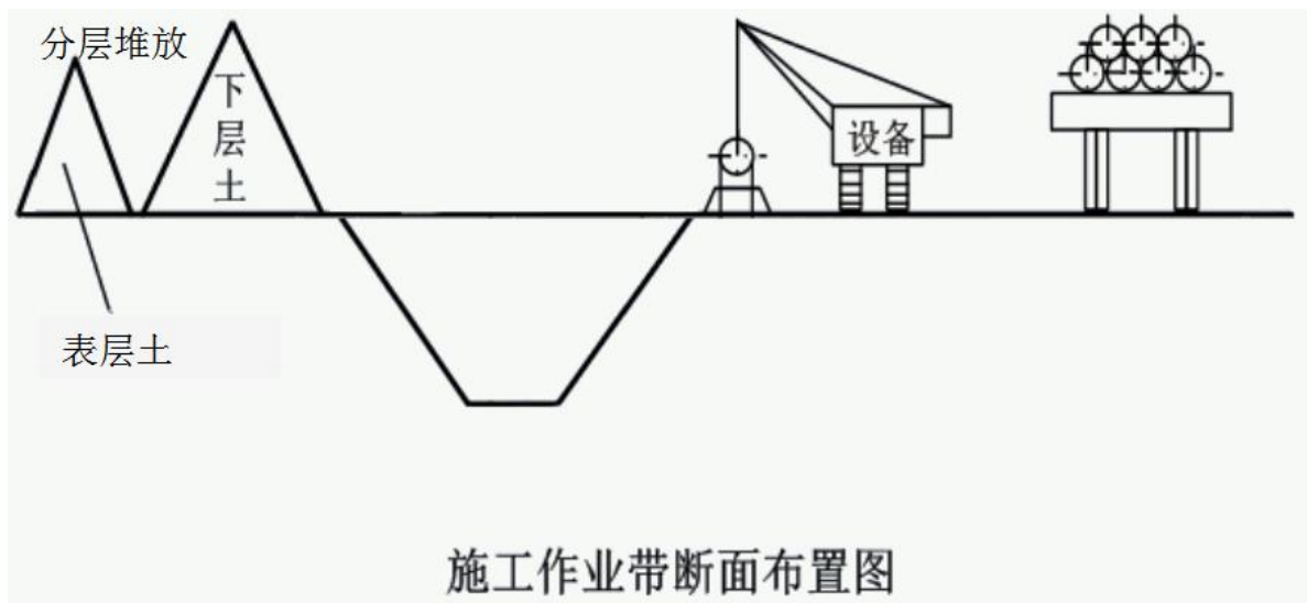
图 3.3-4 一般地段管道施工方式断面示意图
